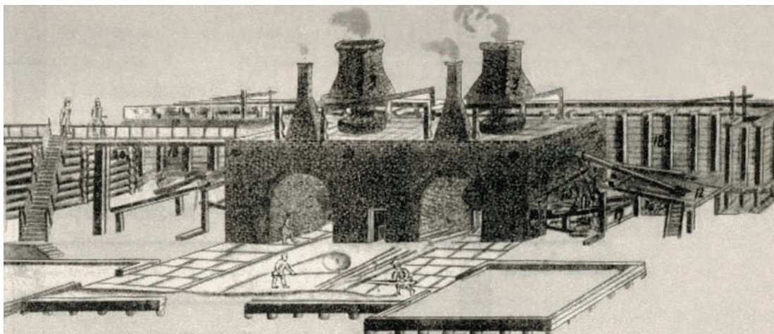
Доменные печи. С рисунка XVIII в. НМ РТ.
